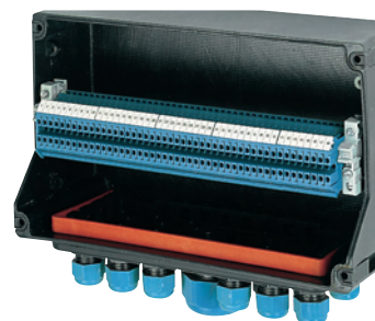
CEAG Sicherheitstechnik GmbH Ex i - Junction Box
